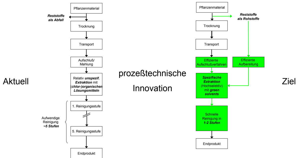
Abbildung 3.3: Strategien der innovativen Phytoextraktion im Rahmen der Nutzung nachwachsender Rohstoffe (grün: Effizienzsteigerung durch verbesserte Aufschluß-/Aufbereitungsverfahren, hochselektive Extraktionstechniken und integrierte Reinigungsverfahren von Wirkstoffen).
